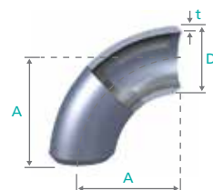
CODO 90° RADIO LARGO
